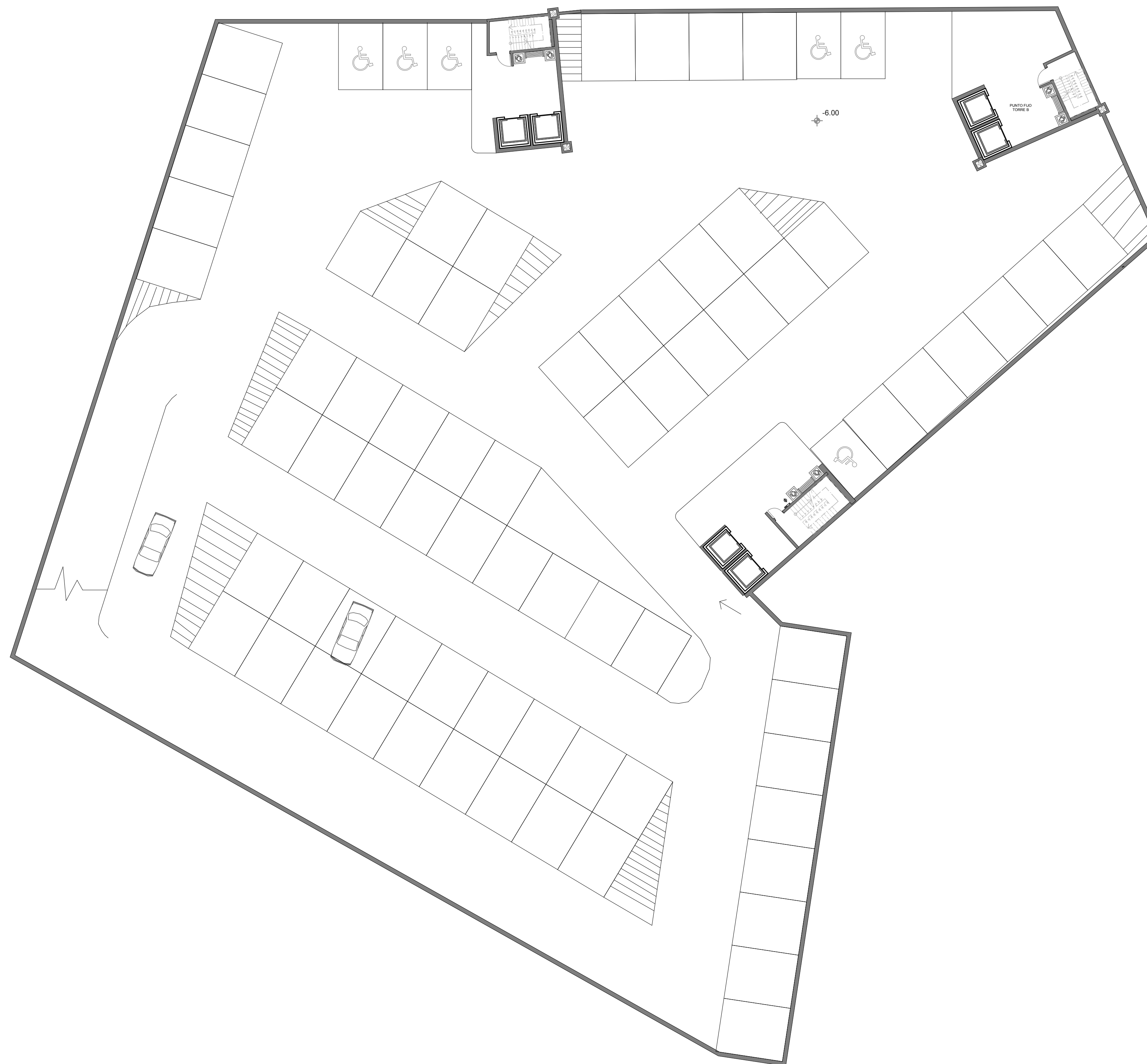
A2 PLANTA DE PARQUEADEROS NIVEL 2 ESCALA 1:200
