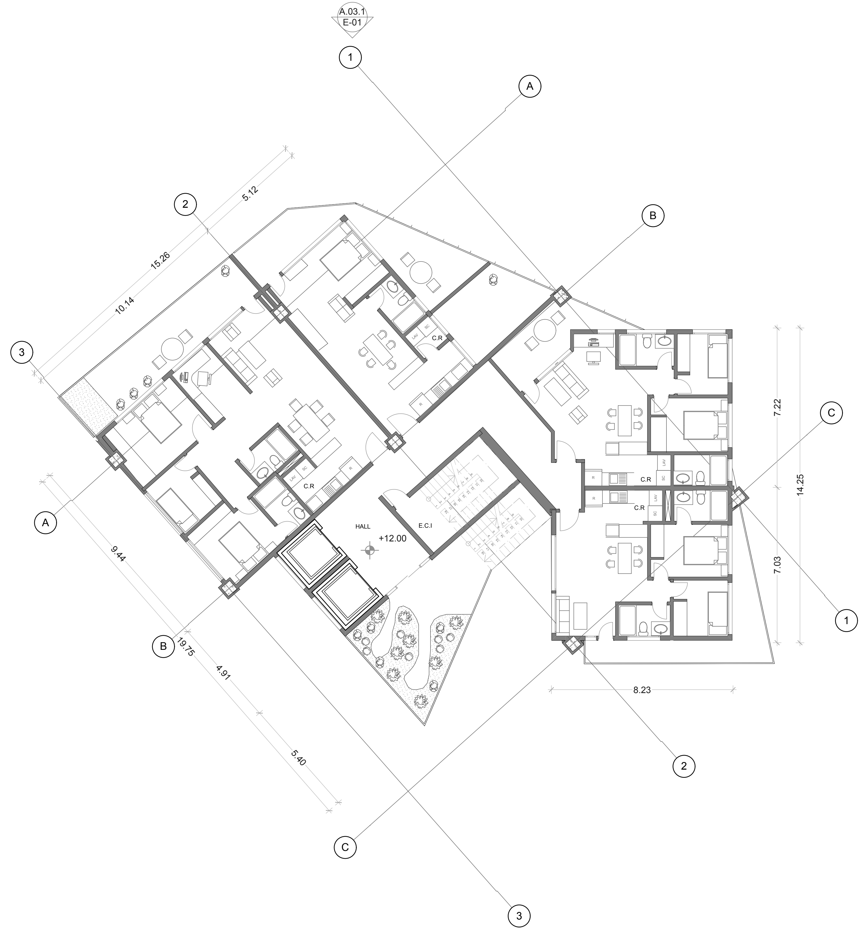
A1 PLANTA VIVIENDA TORRE B PISO 4 ESCALA 1:100
