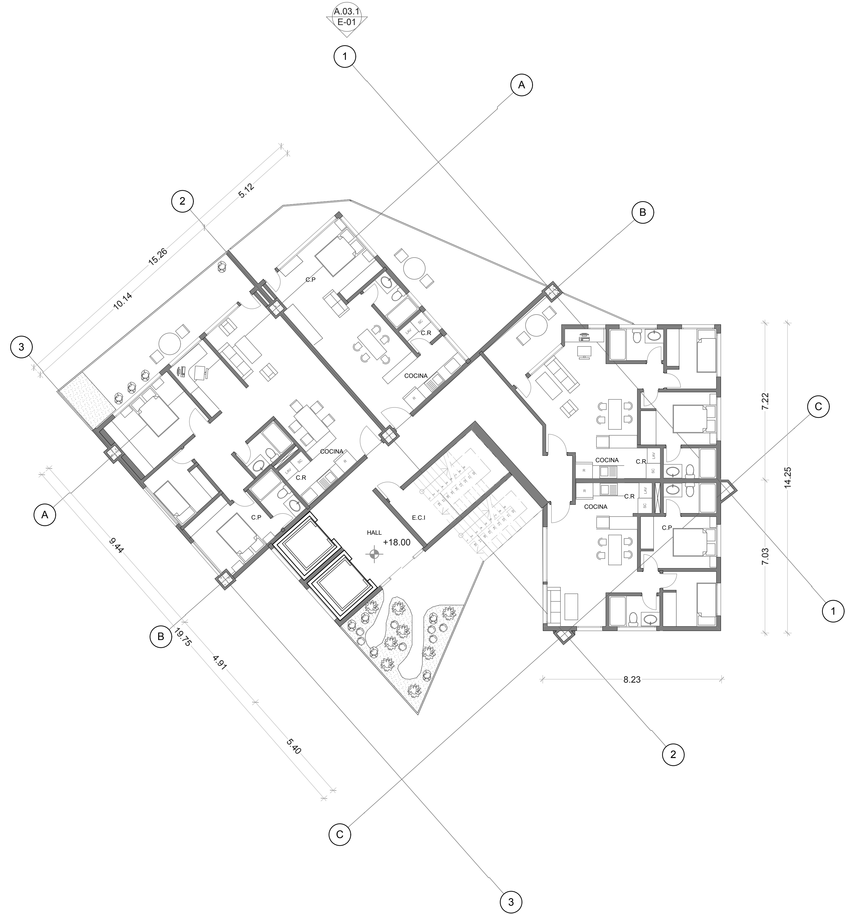
A3 PLANTA VIVIENDA TORRE B PISO 6 ESCALA 1:100
