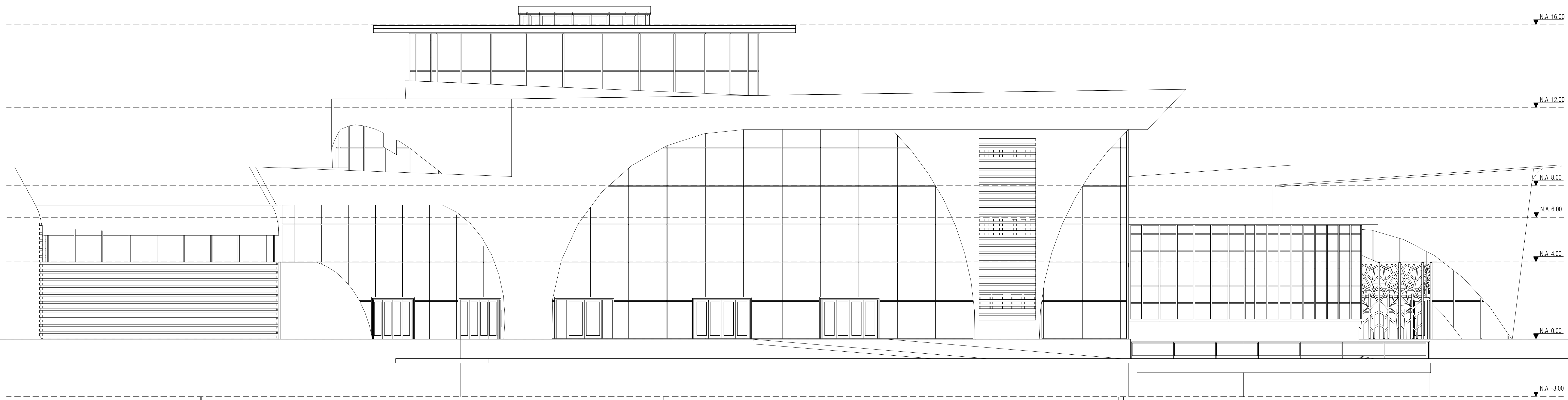
FACHADA SUR ESCALA: 1:100
