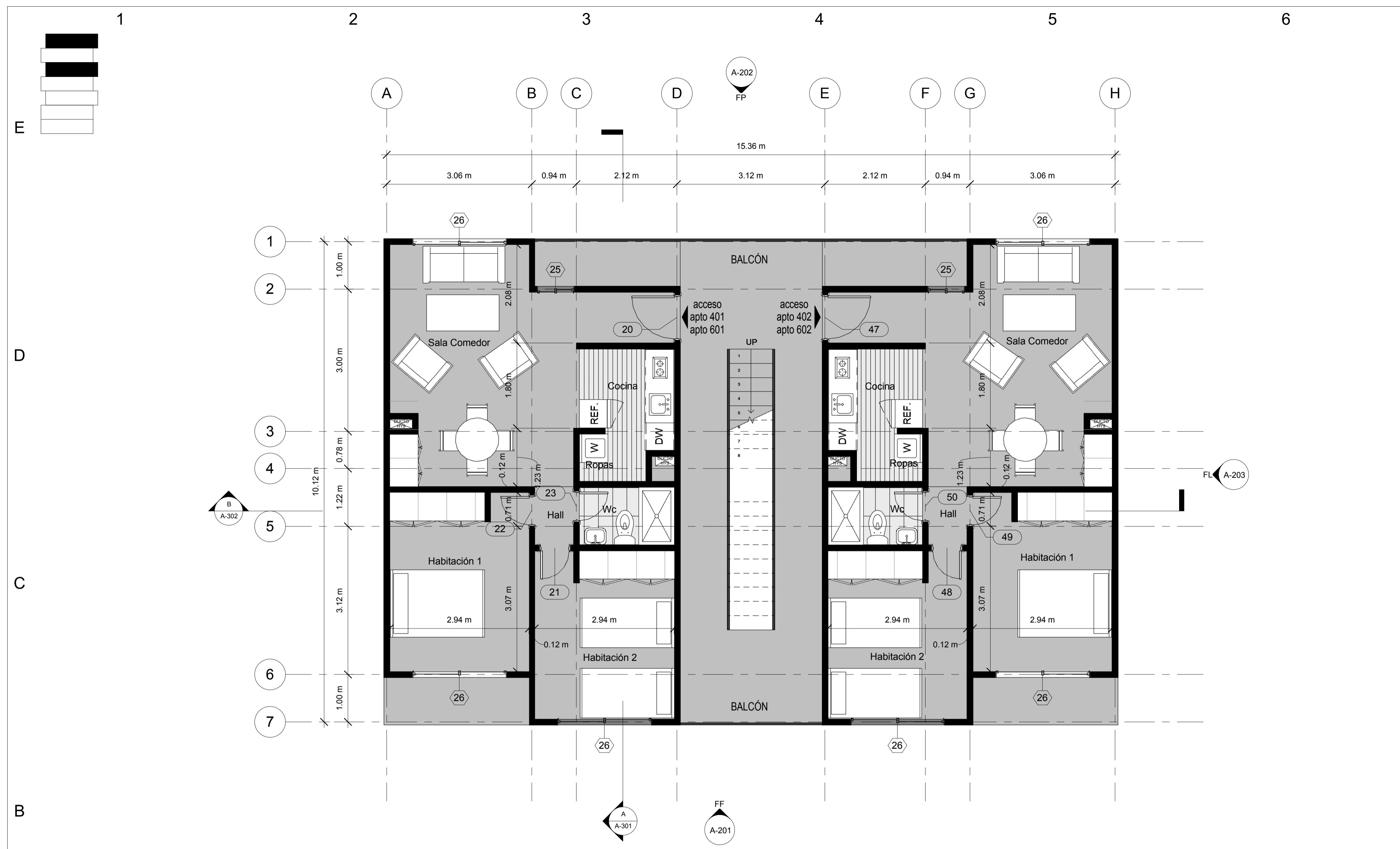
1 Planta 4 Bloque 54 1:50
