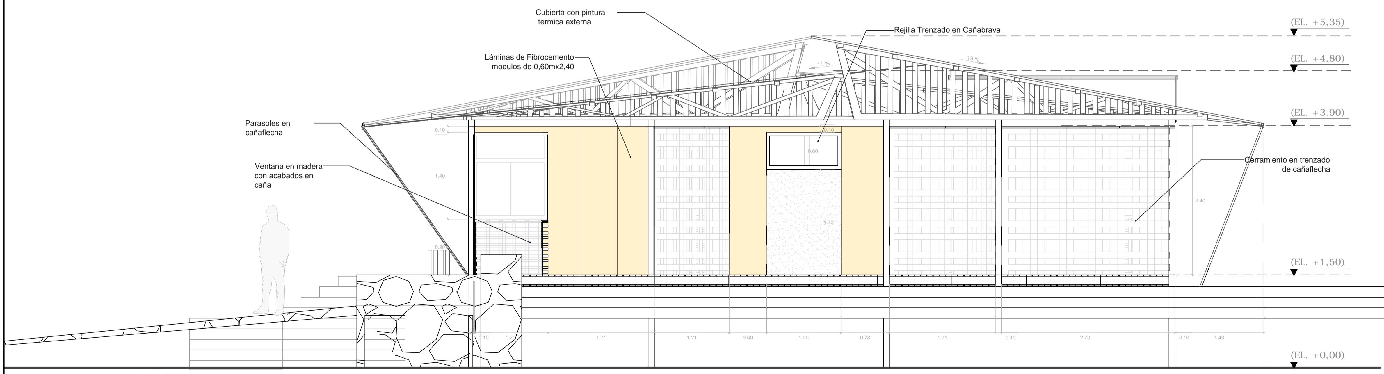
F3 FACHADA LATERAL IZQUIERDA ESCALA 1:20
