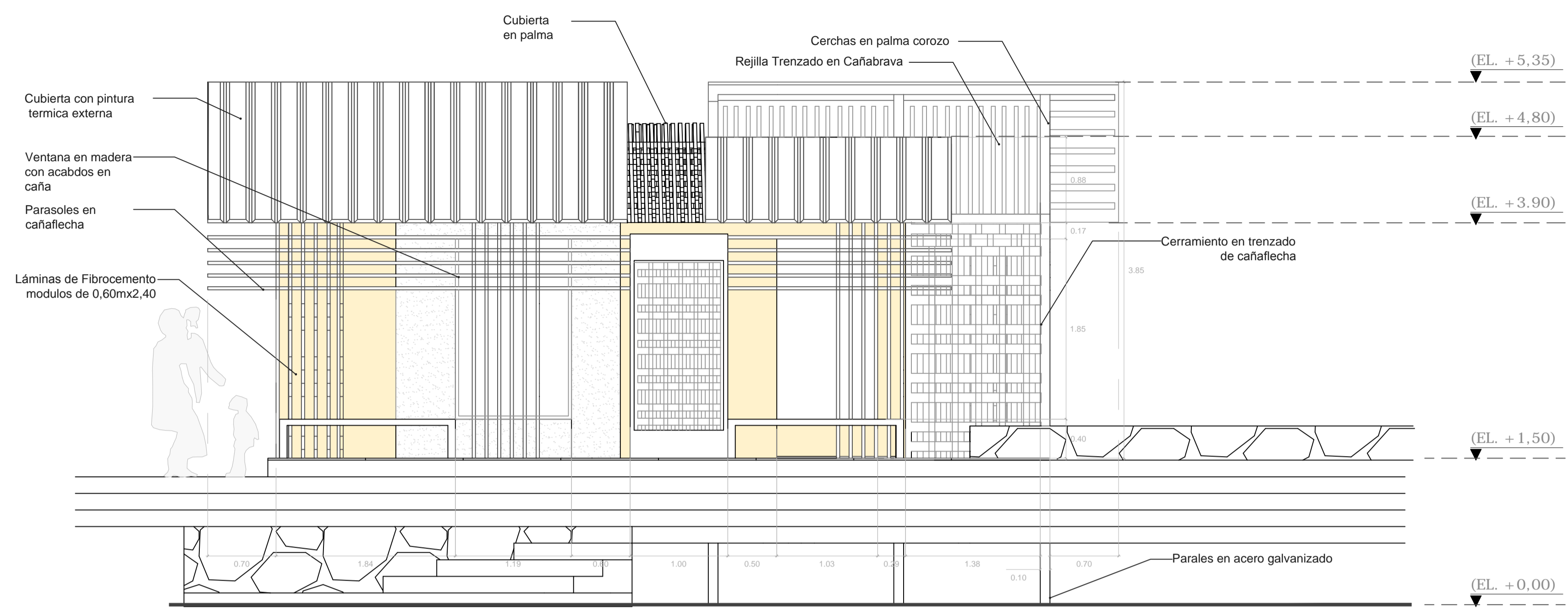
F1 FACHADA PRINCIPAL ESCALA 1:20
