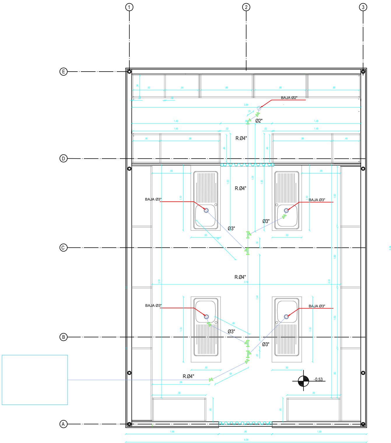
PLANTA DESAGUE DE COCINA
