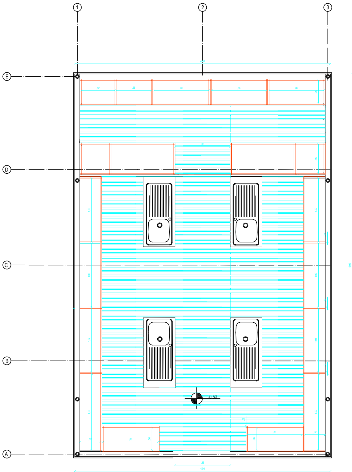
PLANTA DE COCINA
