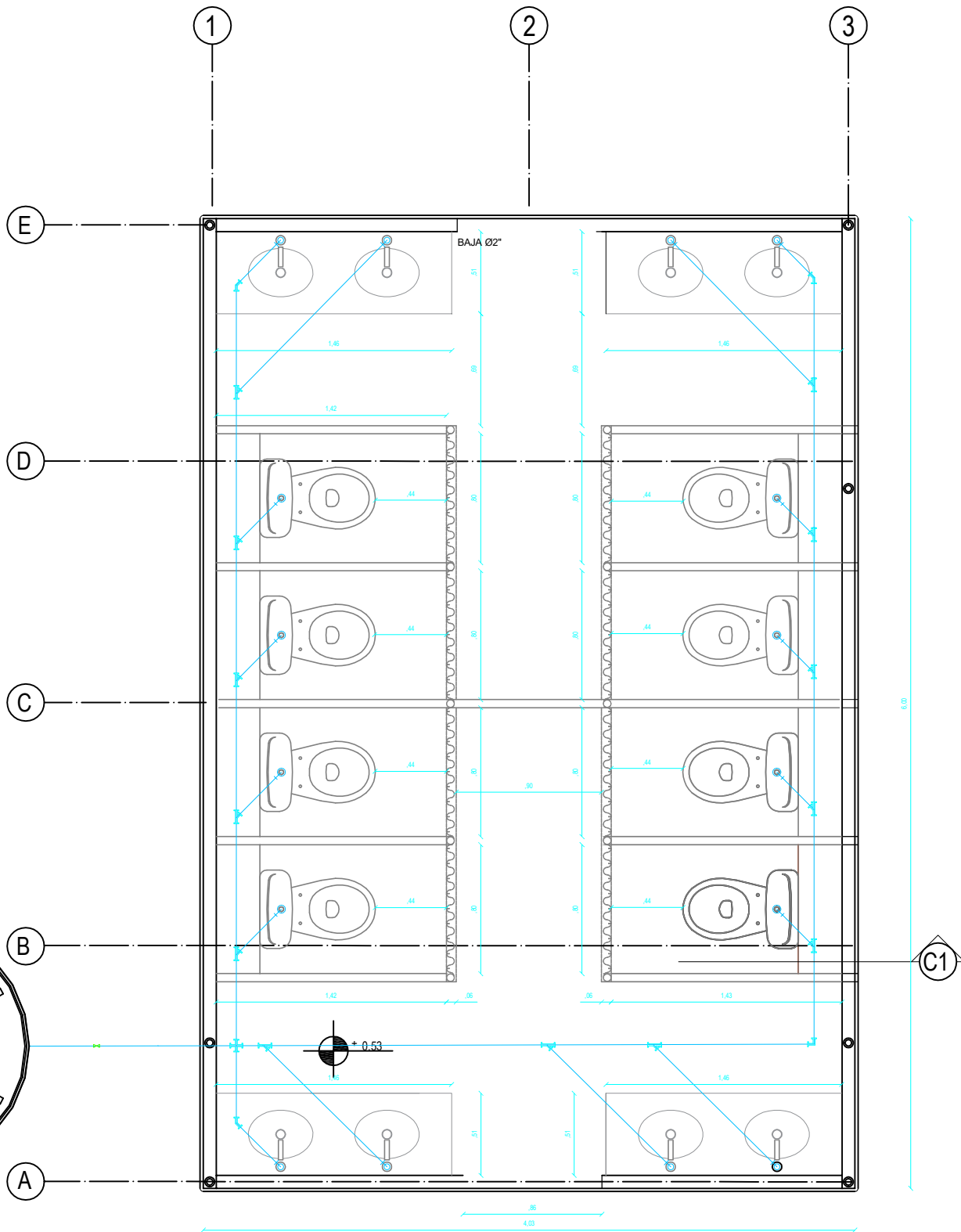
PLANTA ABASTECIMIENTO
