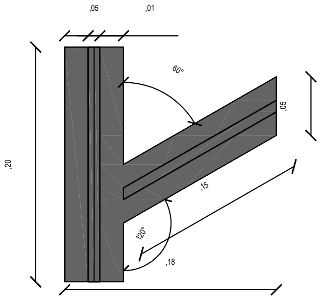
C1 Detalle Alzado Esc: 1:1
