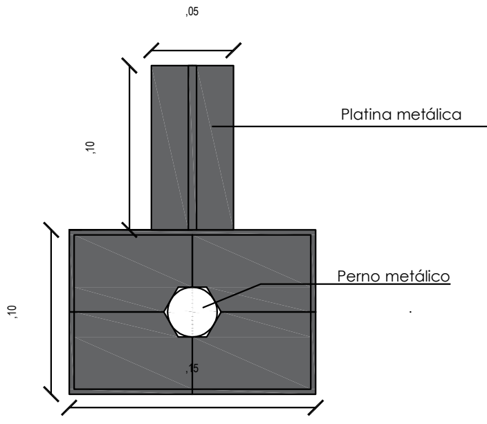
C1 Detalle Alzado Esc: 1:1
