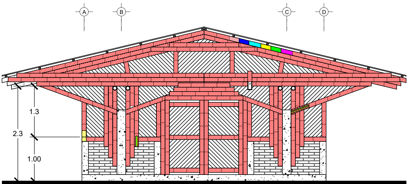
FACHADA ESTE
