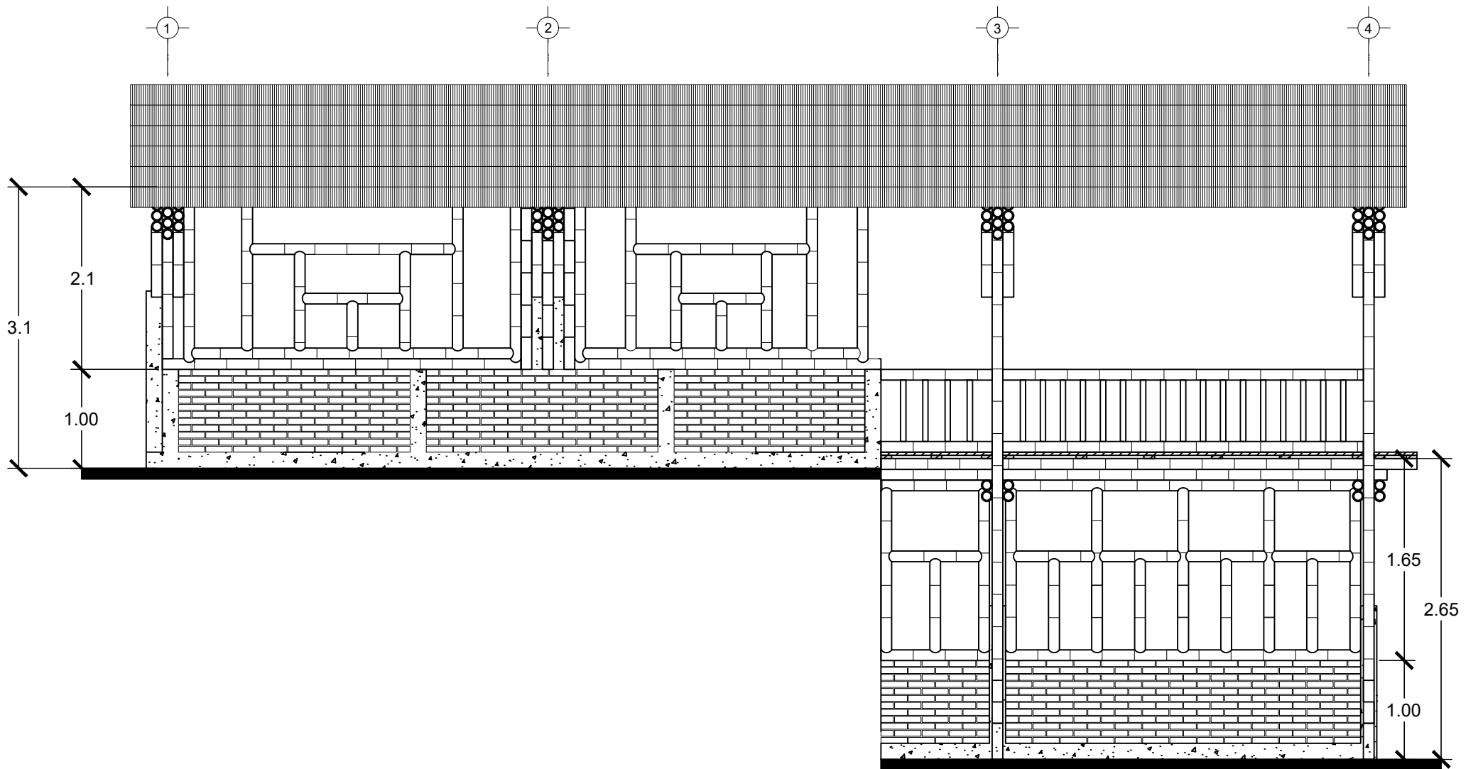
FACHADA NORTE
