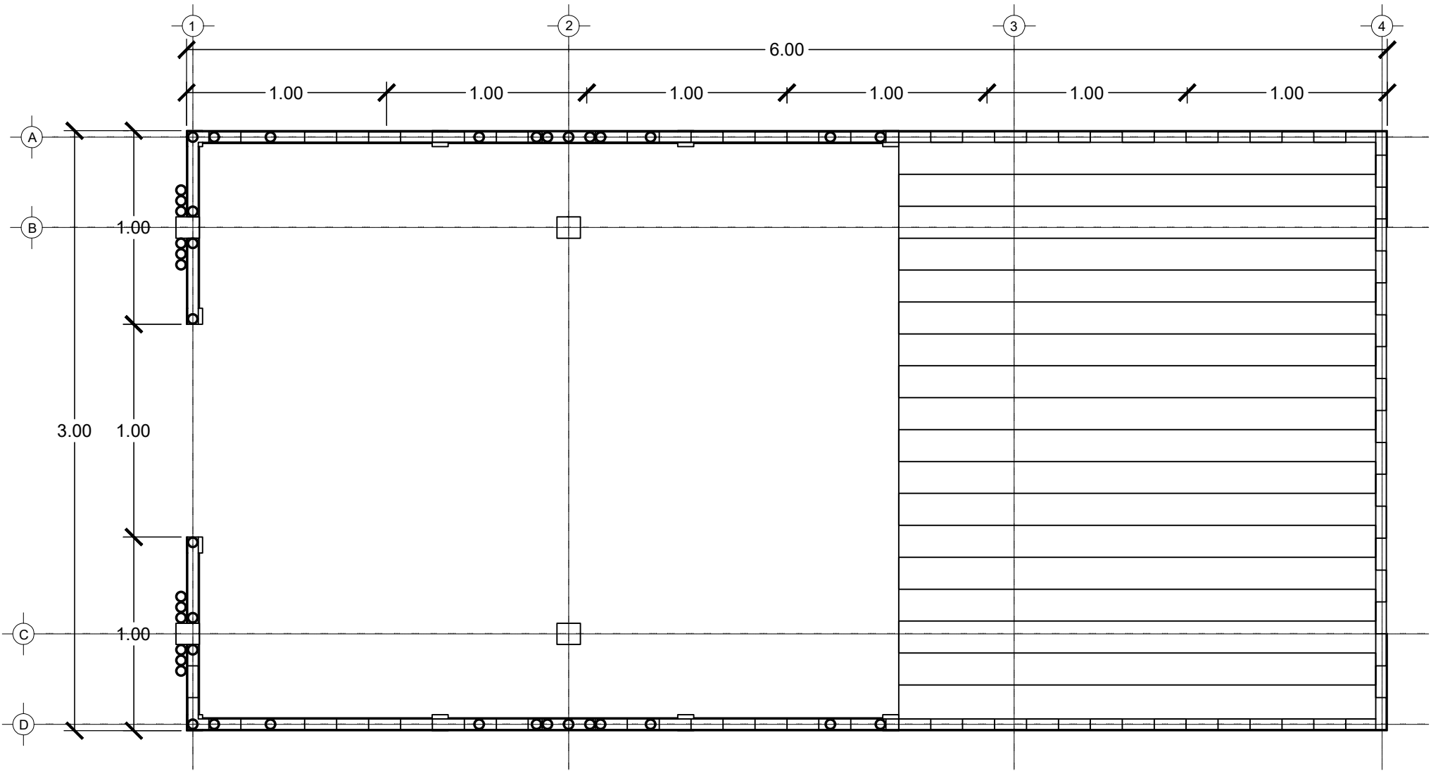
PLANTA NIVEL 2
