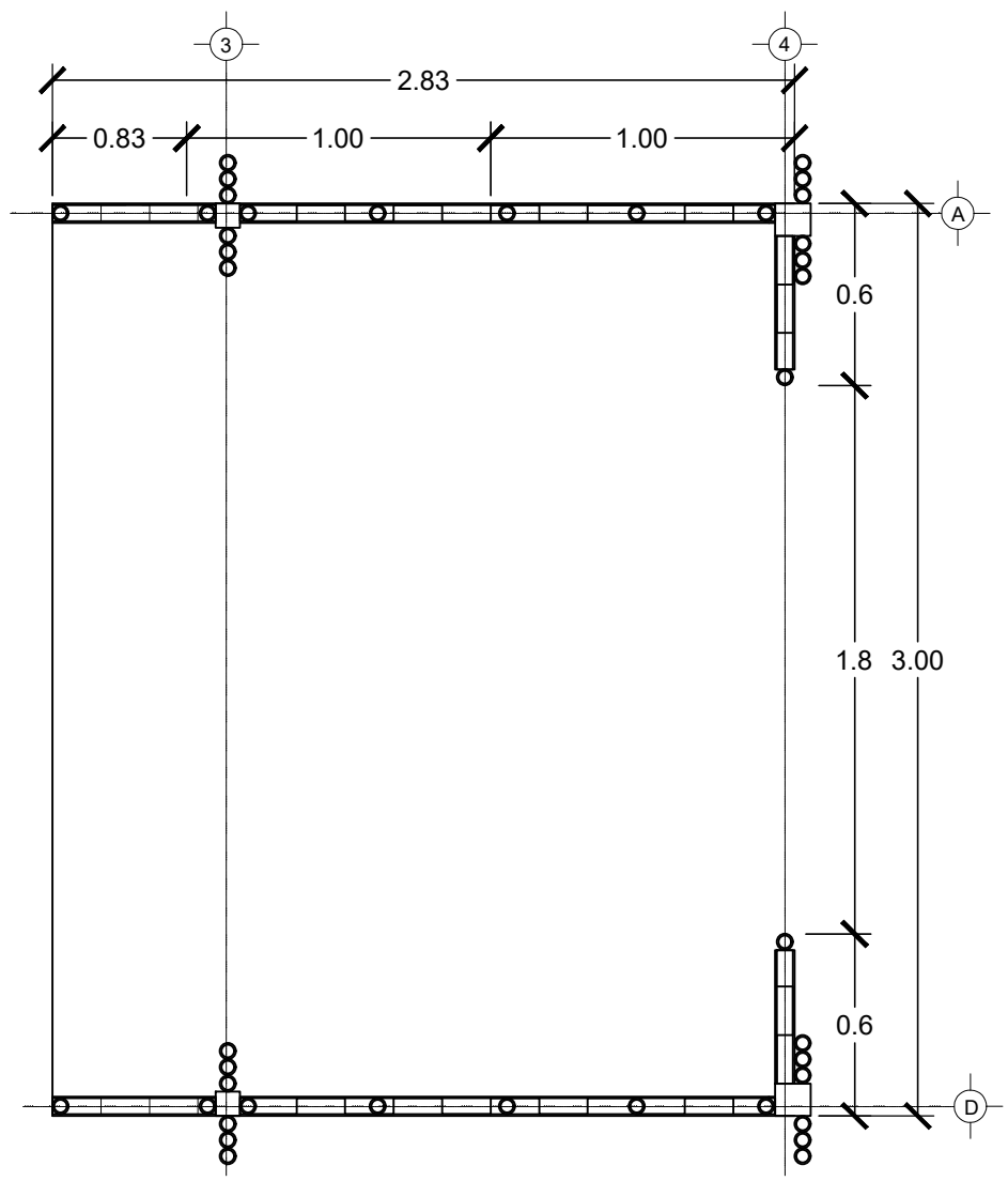
PLANTA NIVEL 1
