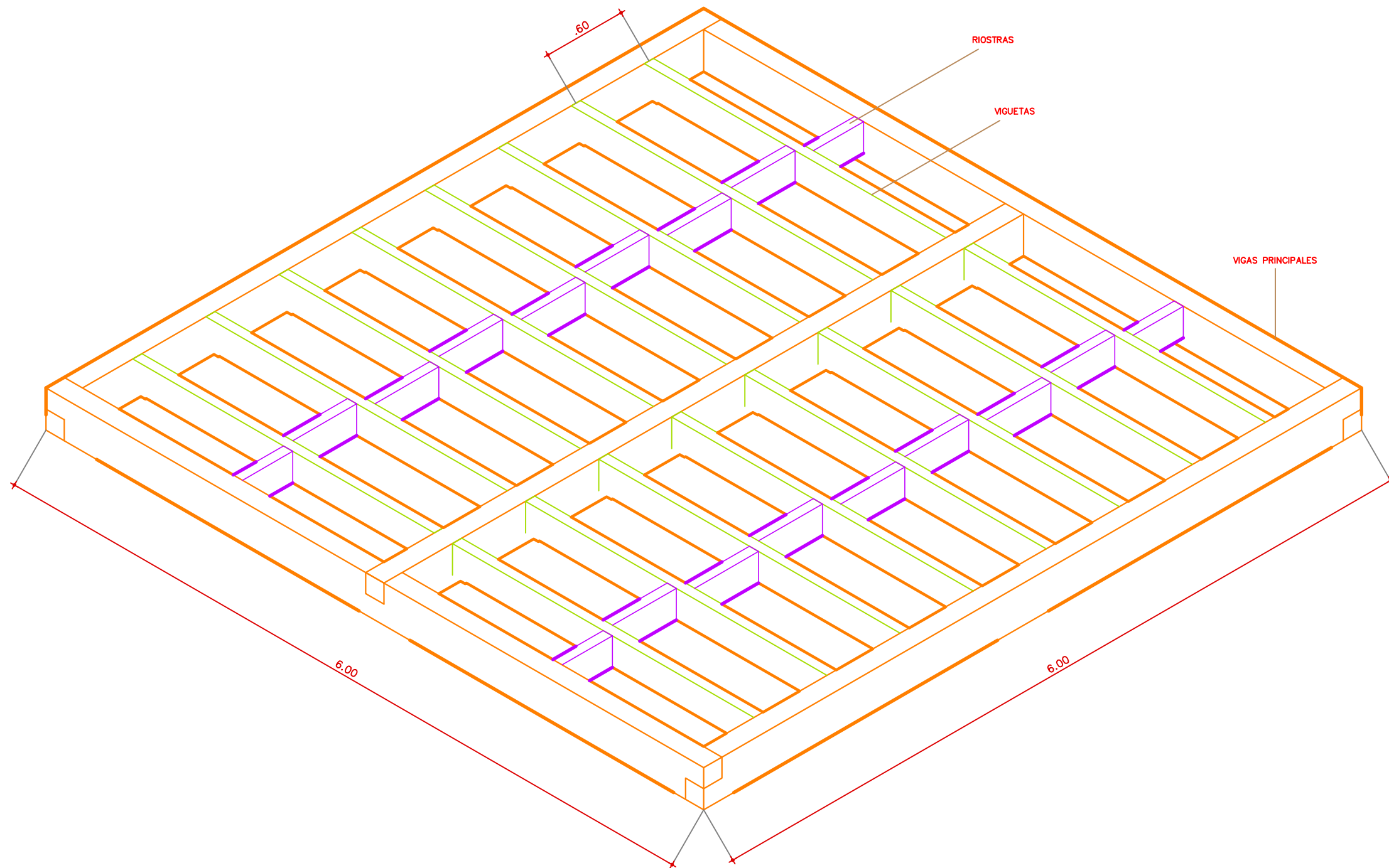
ENTRAMADO PARA ENTREPISO DE 6.00m X 6.00m NOMBRE DE PLANTA
