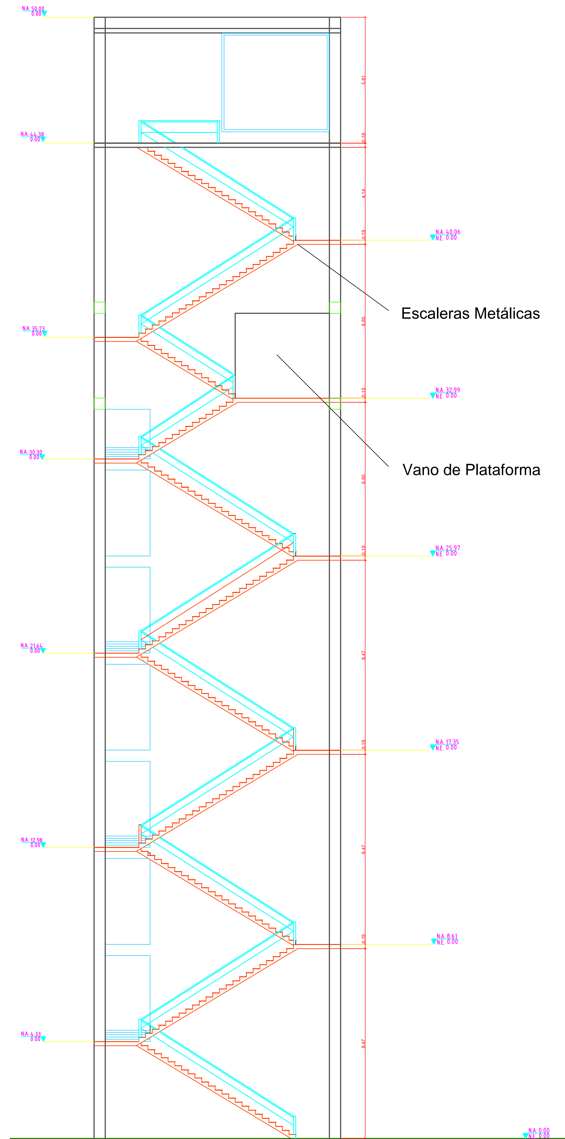
CORTE TRANSVERSAL
