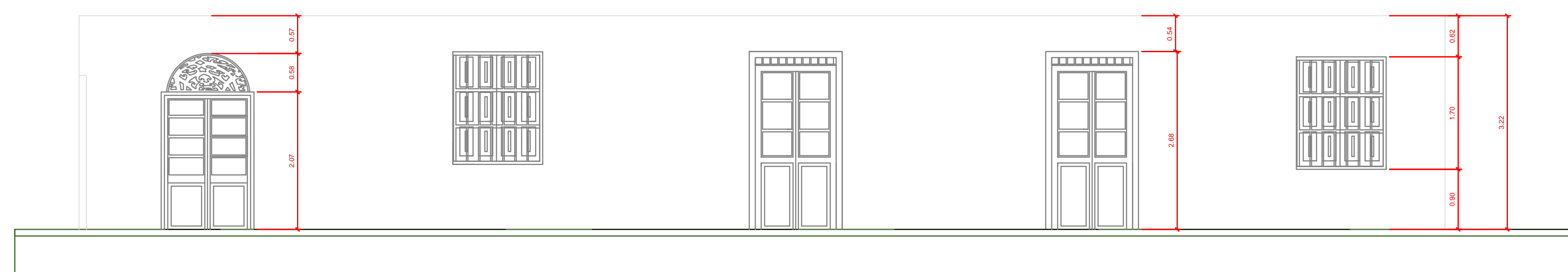
FACHADA N° 5
