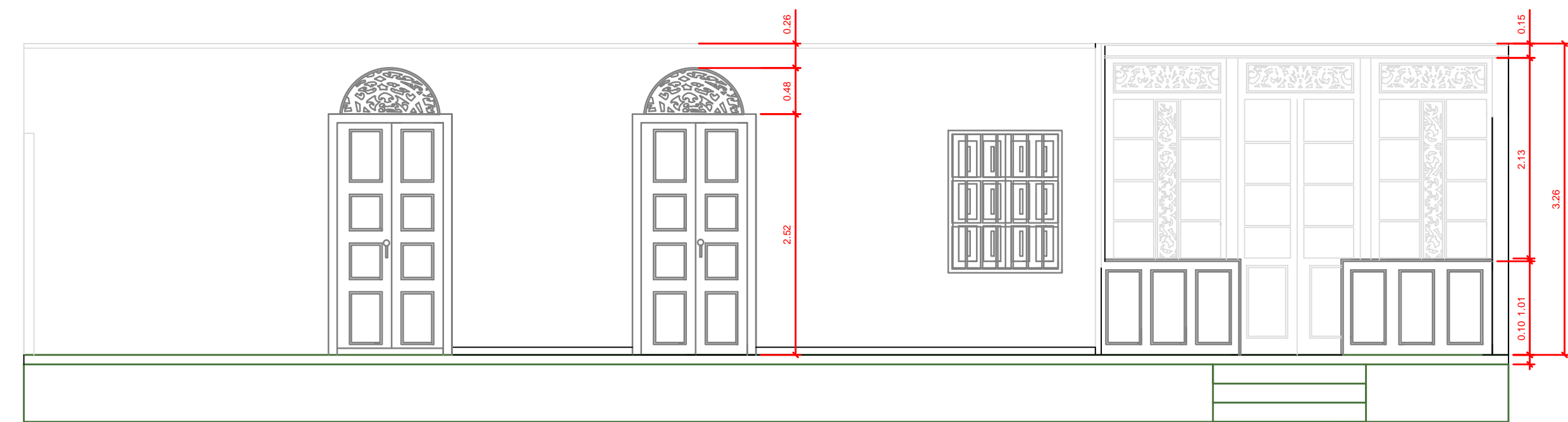
FACHADA N° 1
