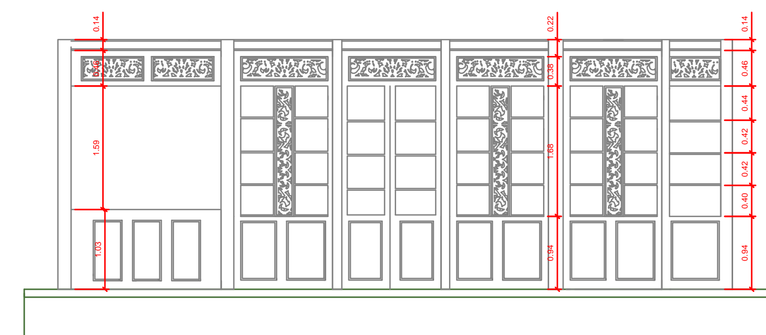
FACHADA N° 4
