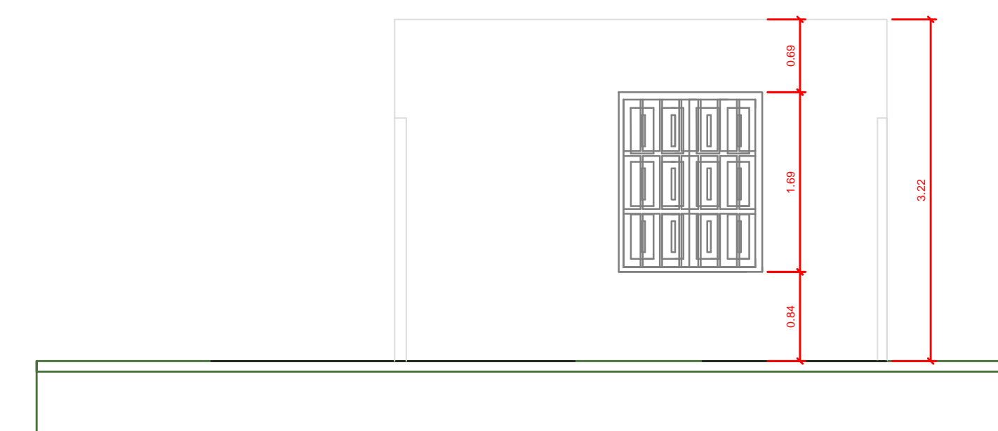
FACHADA N° 8
