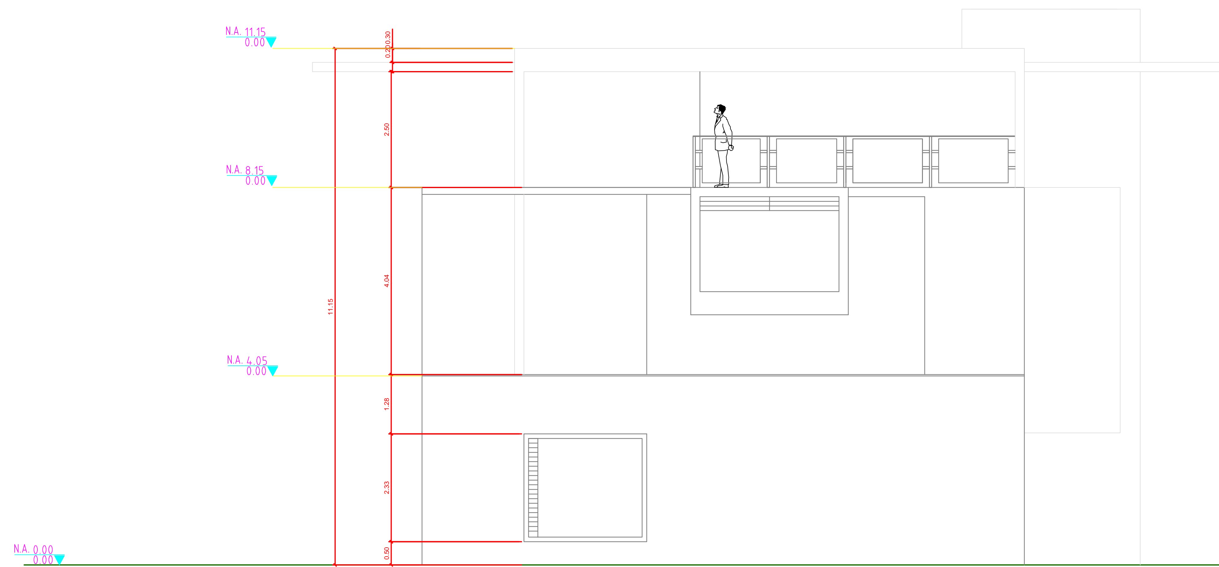
FACHADA LATERAL
