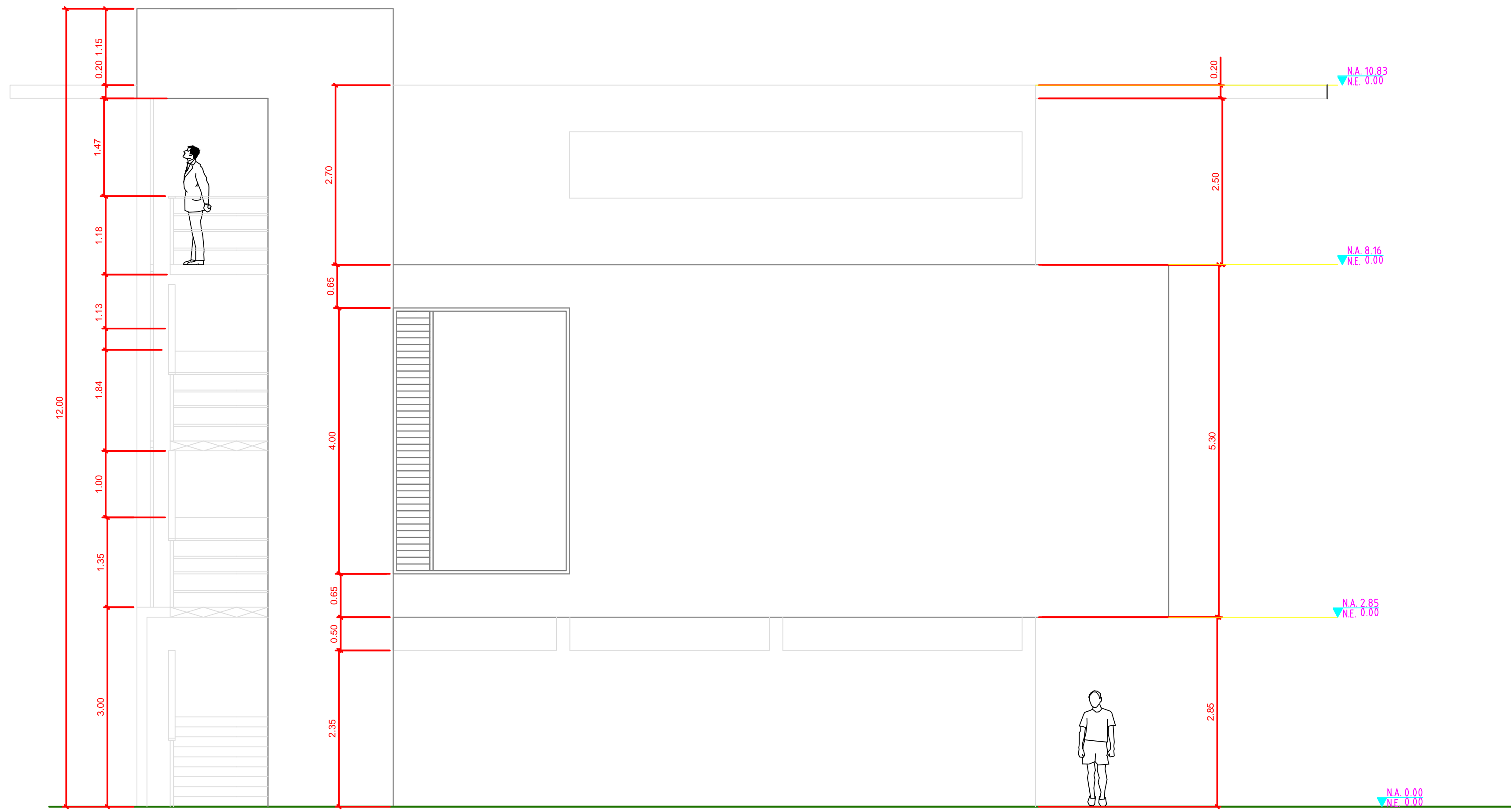
FACHADA FRONTAL
