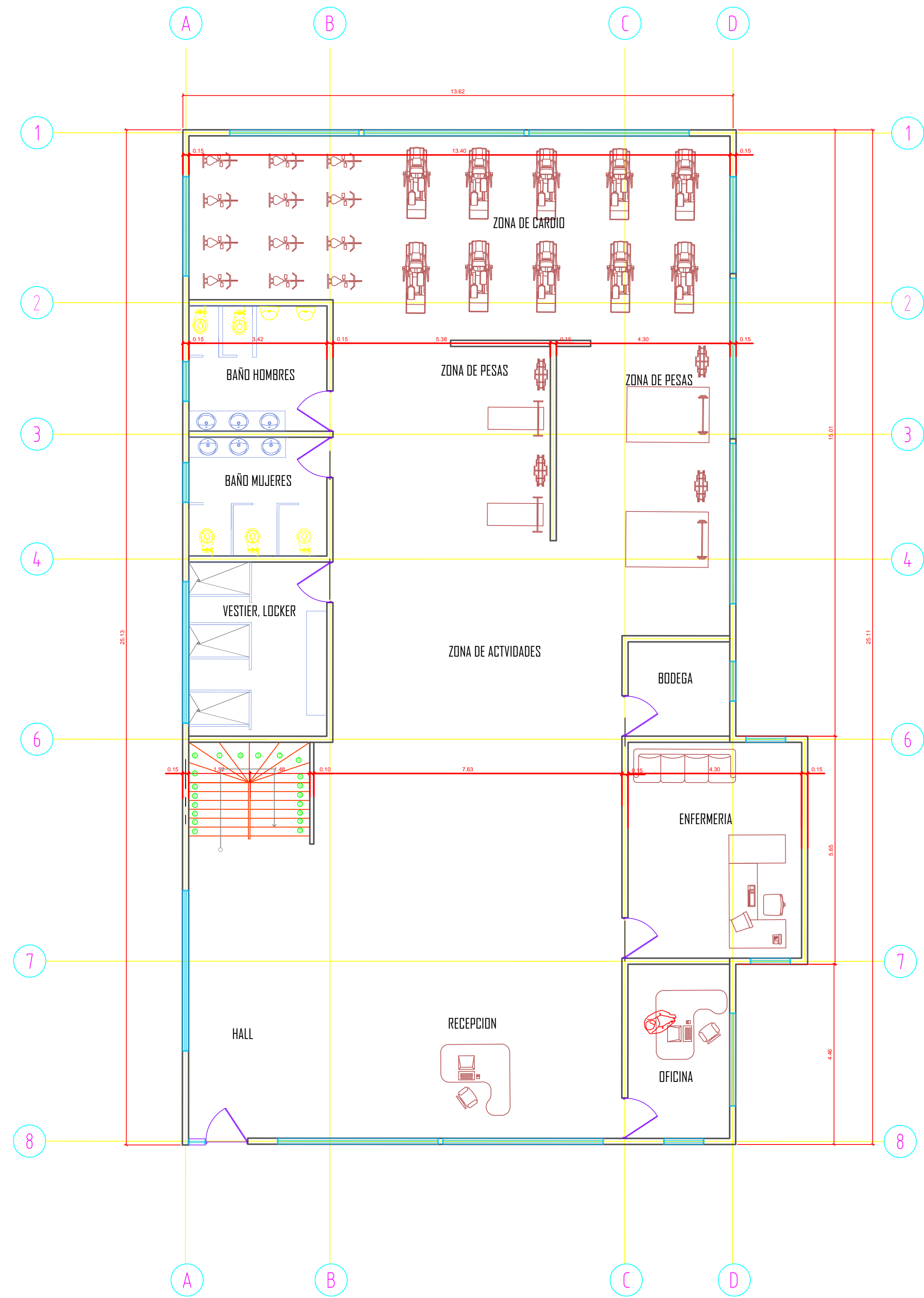
PLANTA PRIMER PISO GIMNASIO
