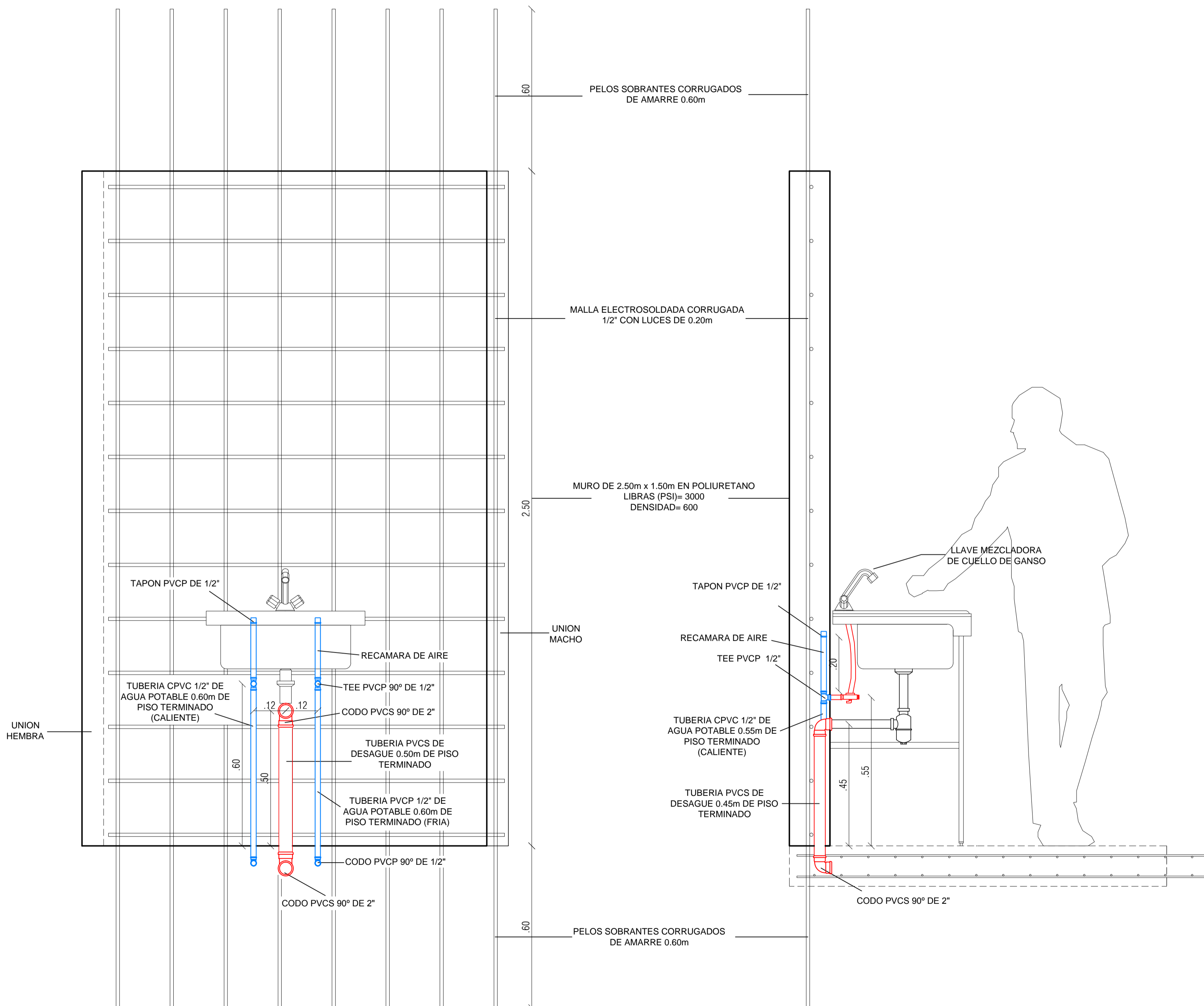
VISTA LATERAL
