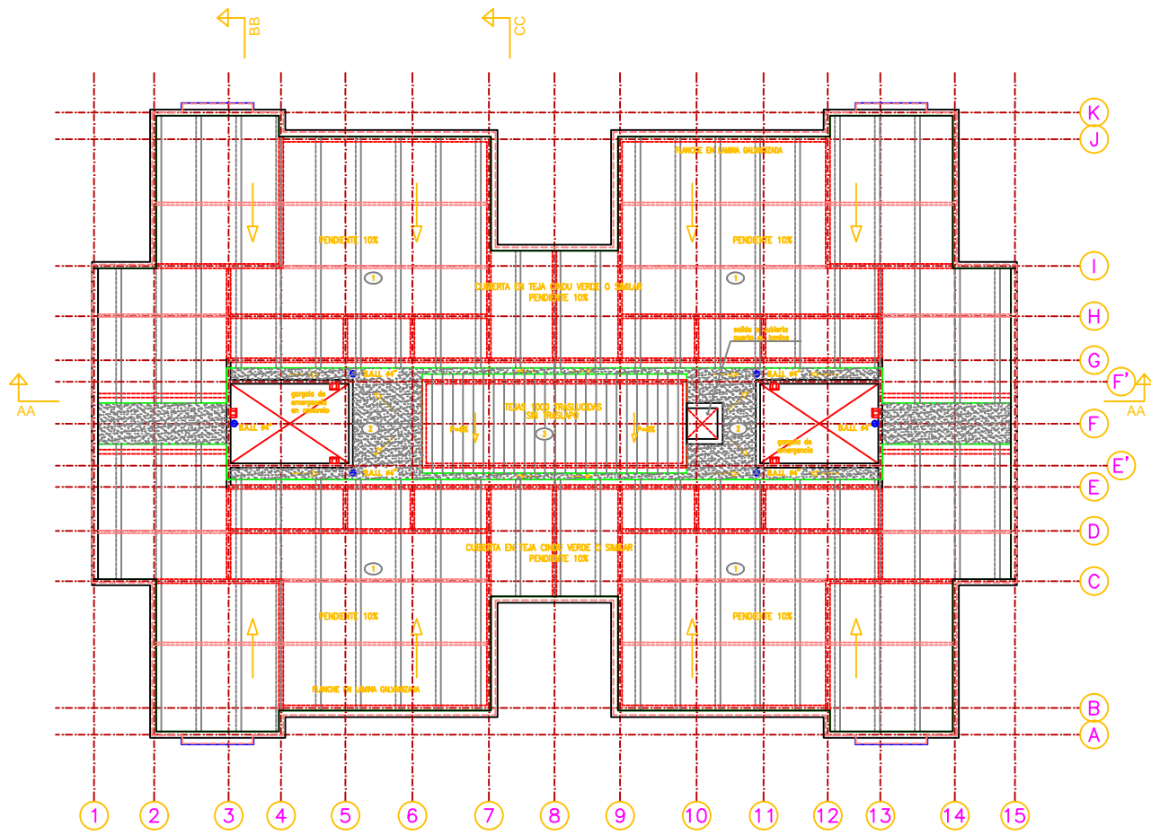
TORRE TIPO PLANTA DE CUBIERTA
