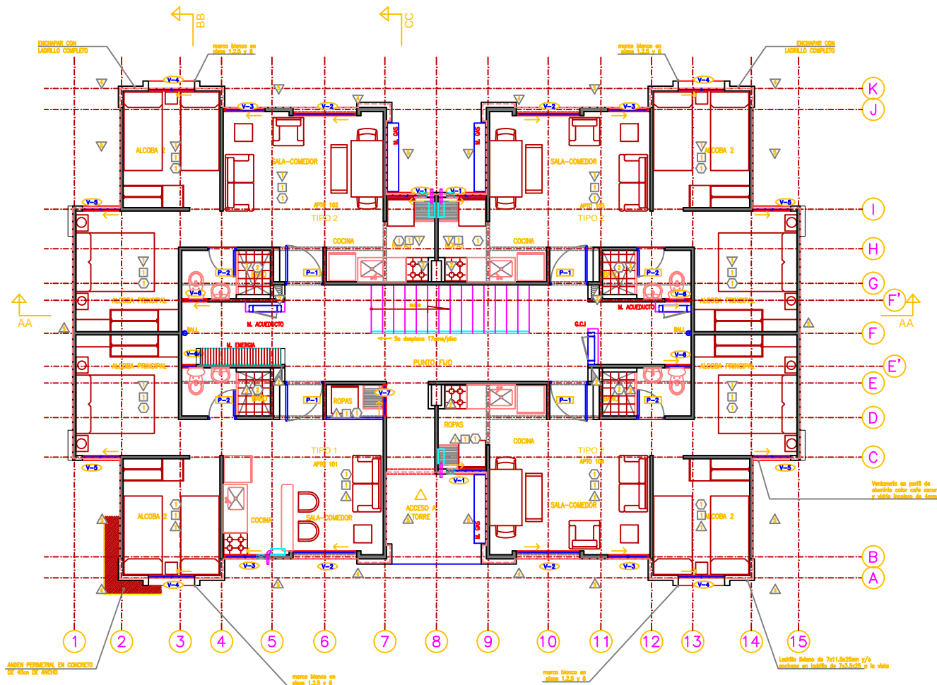
TORRE TIPO PLANTA PRIMER PISO AREA APTO TIPO 1 = 37.27 M2 AREA APTO TIPO 2 = 40.12 M2
